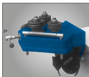
Horizontální pracovní poloha se sklopenou hlavou stroje
