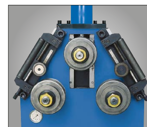
Speciální boční vodící kladky pro úhlové zakružování
