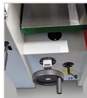
▶ Výškové přestavení stolu pomocí ručního kola
